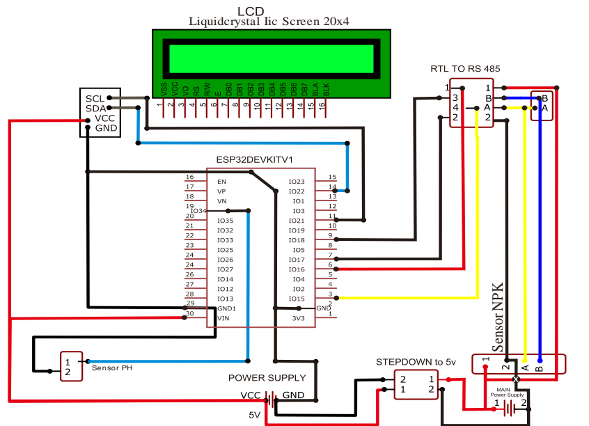
Gambar 4. Skema Rangkaian Alat Monitoring pH dan NPK Kompos Tandan Kosong Kelapa Sawit
