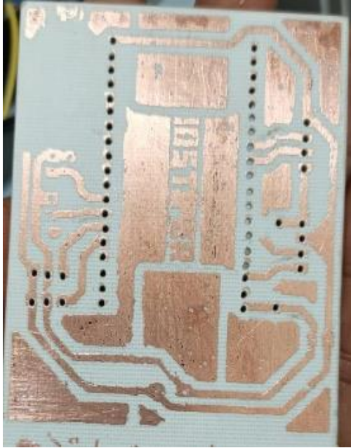
Gambar 7. Hasil Cetak Manual PCB
