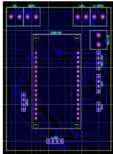
Gambar 6. Papan Sirkuit Sebelum Cetak
