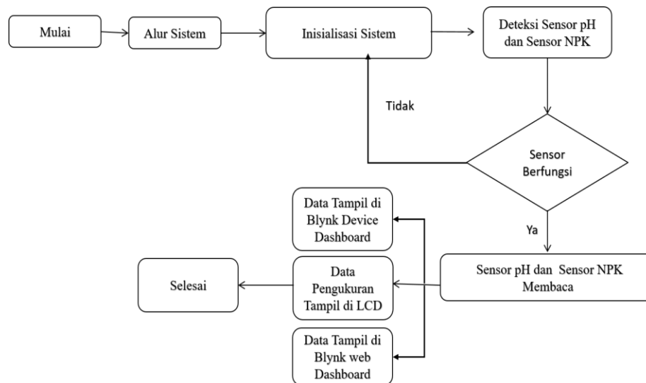
Gambar 7. Alur Kerja Perangkat Lunak (Software)
