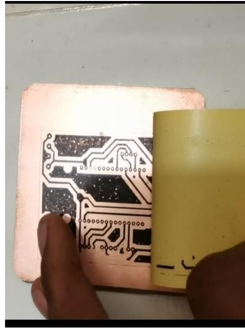
Gambar 8. Proses Pemindahan jalur PCB
