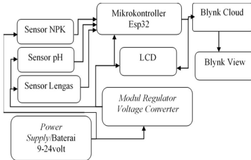
Gambar 3: Diagram Sistem Kerja Alat Monitoring pH dan NPK
